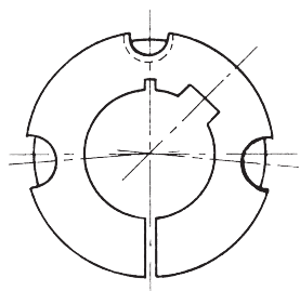
A KIVITEL 3 db rögzítő furattal
